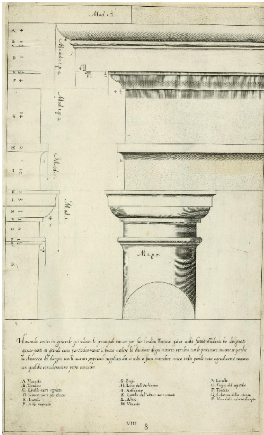
Joonis 89 – Toskaana orderi antablemaan ja kapiteel – Vignola, 1635
