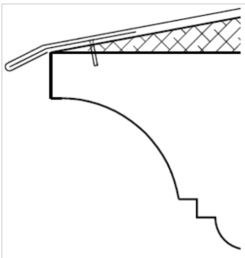
Joonis 39 – Plekiribaga kinnitamine – Muinsuskaitseamet – hooneosade näidislahendused
