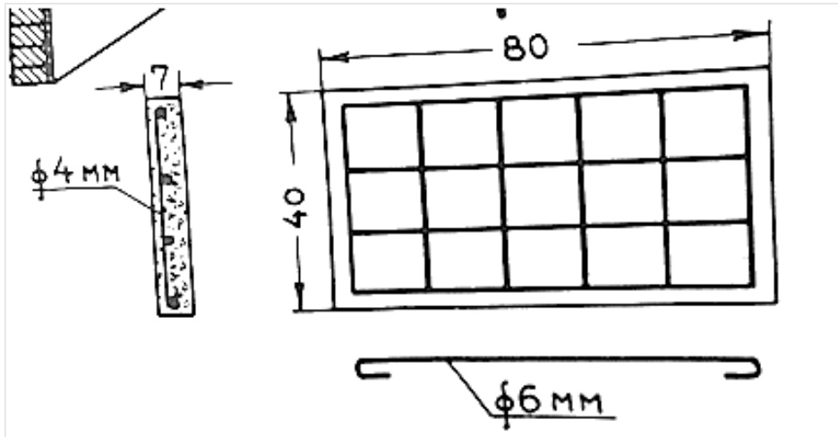
Joonis 73 – sardbetoonest karniisiplaat – Veski, 1939
