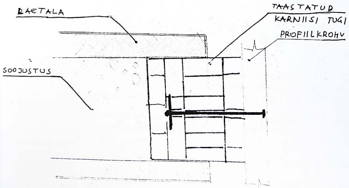
Joonis 46 – Säilinud karniisi kinnitamine ankrutega – Ossip, A. 2012
