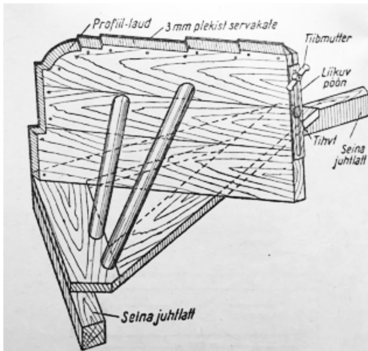
Joonis 41 – Šabloon – Makarov, 1947
