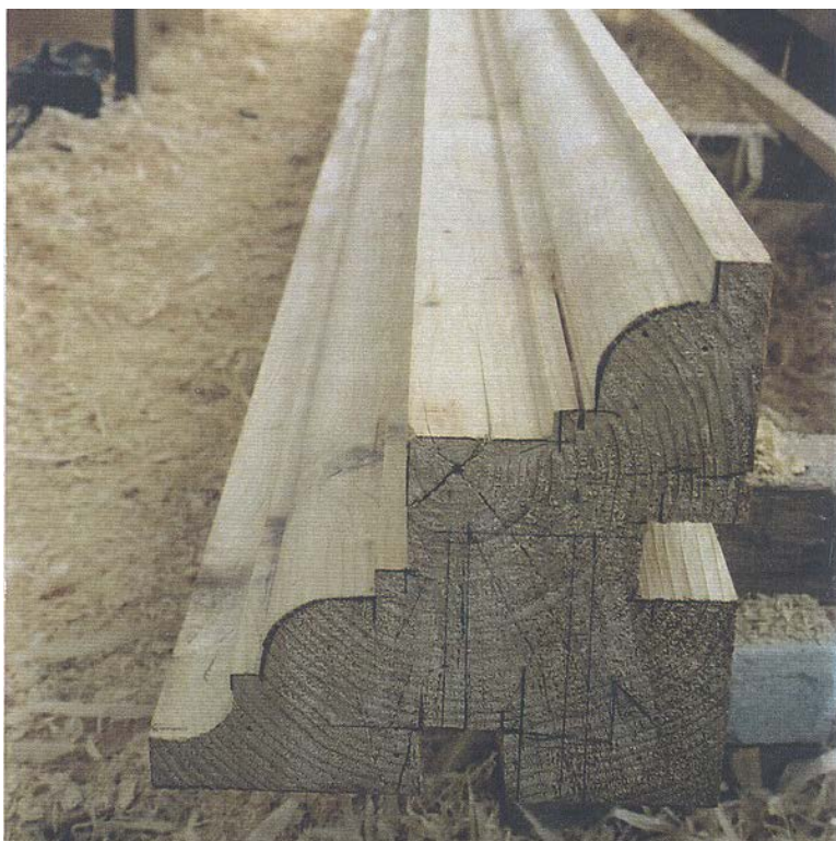
Joonis 78 – Täispuidust karniis – Vali, J. fotokogu
