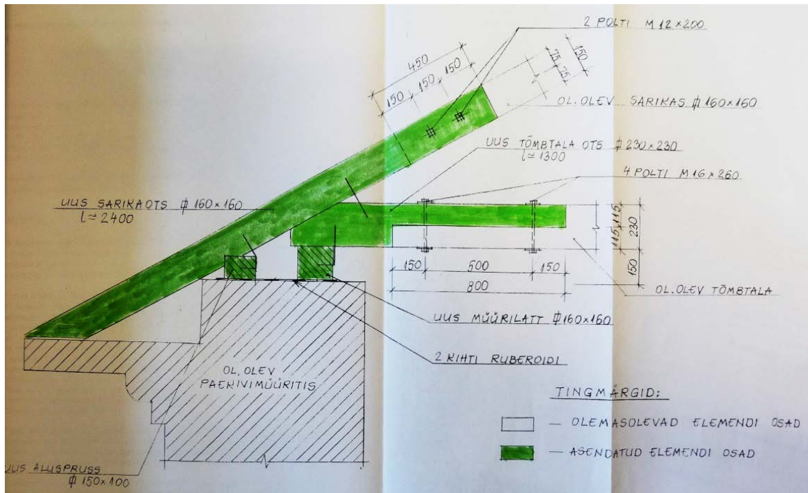
Joonis 70 – Räästasõlme teostusjoonis – Ränd, 1998
