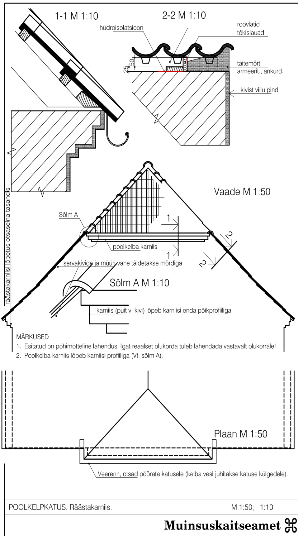
Joonis 95 – Karniis ainult kelbaräästa all – Muinsuskaitseamet – hooneosade näidislahendused
