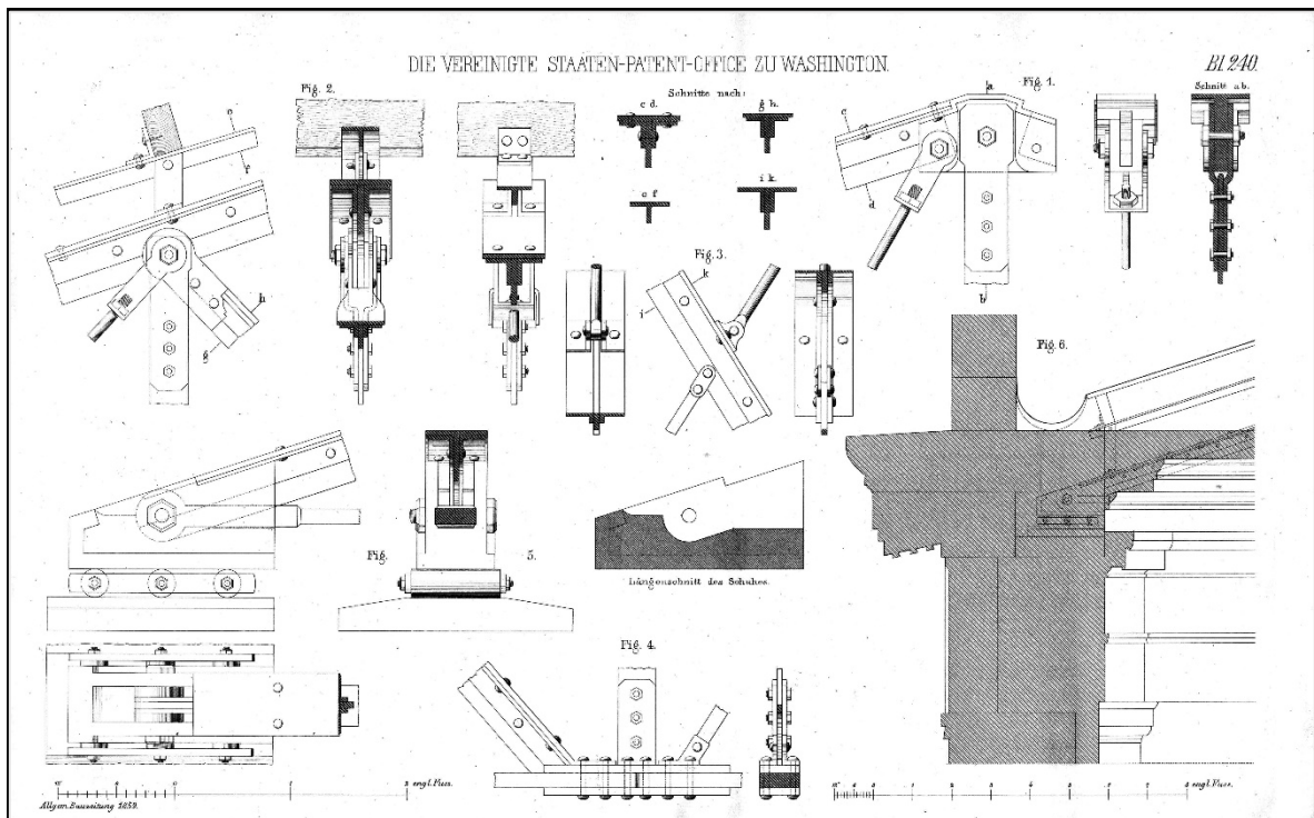
Joonis 20 – Räästalõige ja karniis, patendiameti hoone Washingtonis – Atlas zur Allgemeinen Bauzeitung, 1859
