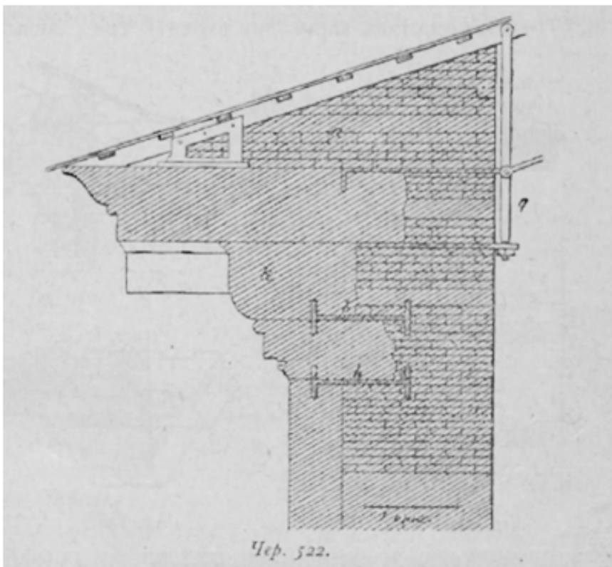
Joonis 22 – Horisontaalsete ankrutega kinnitatud karniis – Романовичъ, 1903
