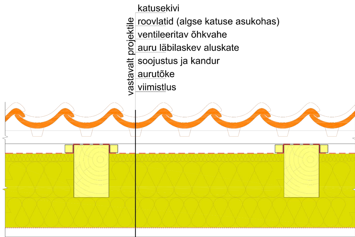
Joonis 84 – Katuse soojustamine alggabriite ületamata – Muinsuskaitseamet - hooneosade näidislahendused
