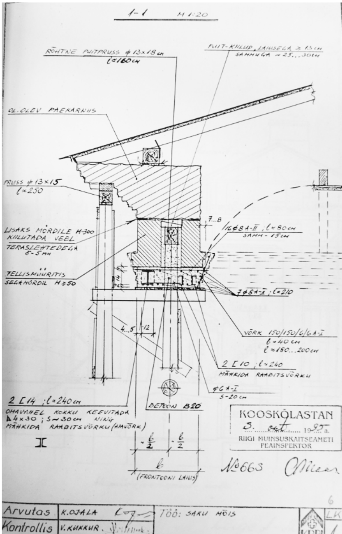
Joonis 67 – Portikuse puitsilluste asendamise lahendus aastast 1995 – Kukkur, 1996
