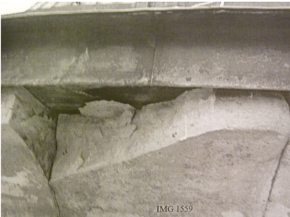
Joonis 56 – Allakukkunud karniisiosa – As Irbistero, 2013, n9.8437
