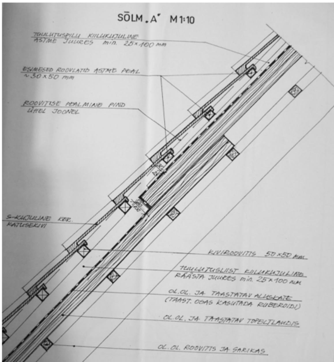
Joonis 87 – 2009. ja 2012. aastal tööde aluseks olnud katuse lõige – Rajari 2009
