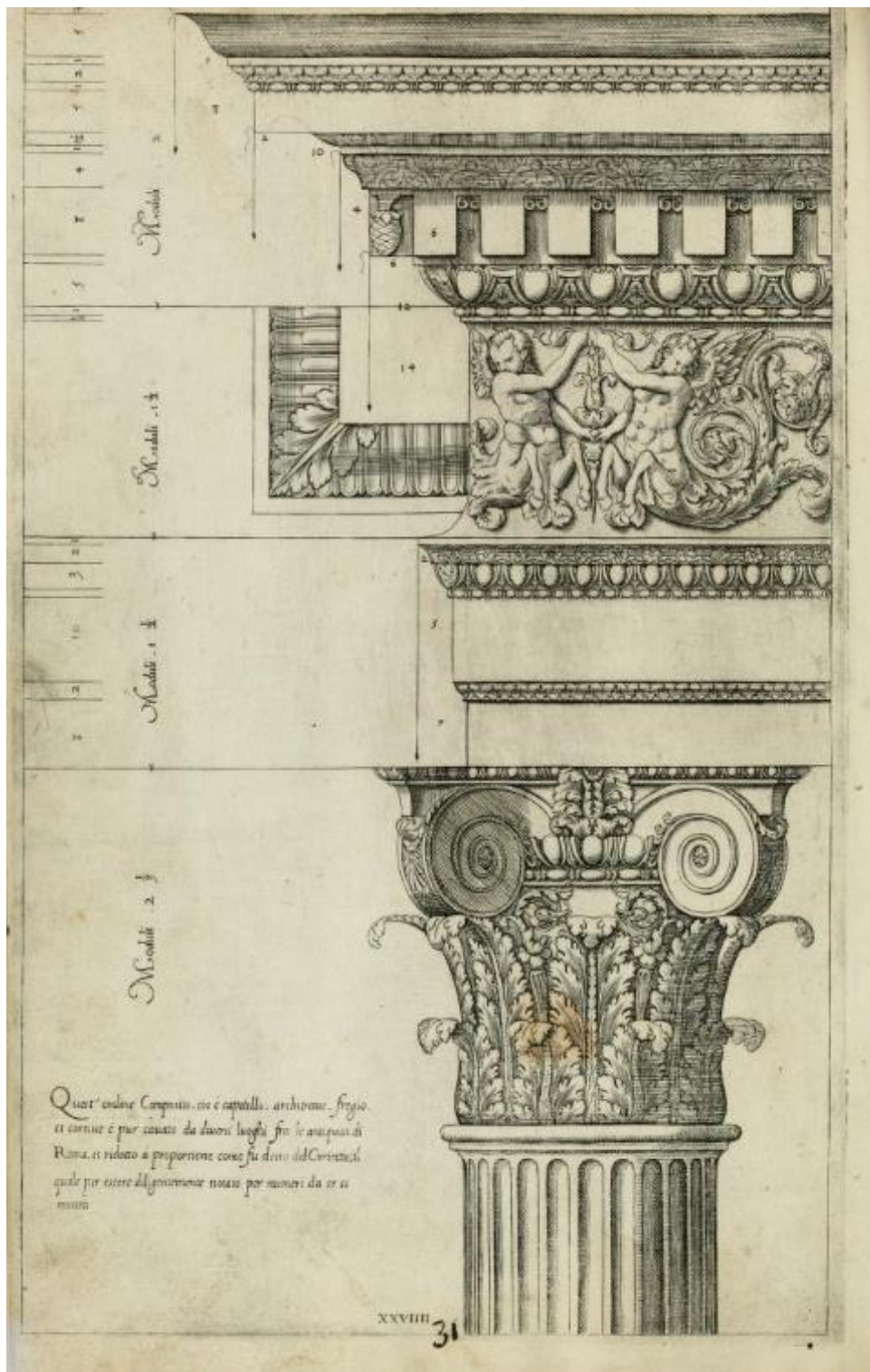
Joonis 93 – Komposiitorderi antablemaan ja kapiteel – Vignola, 1635
