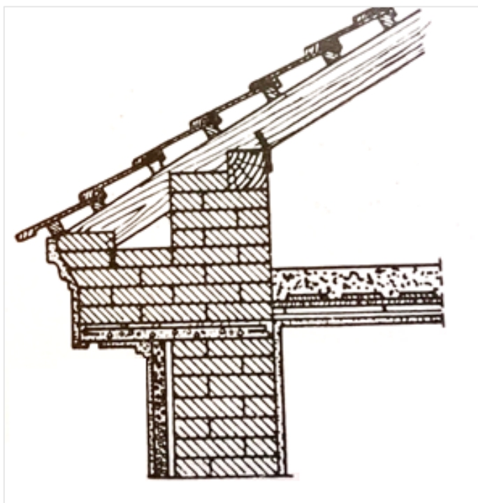
Joonis 72 –Karniis sardbetoonplaadil – Veski, 1939
