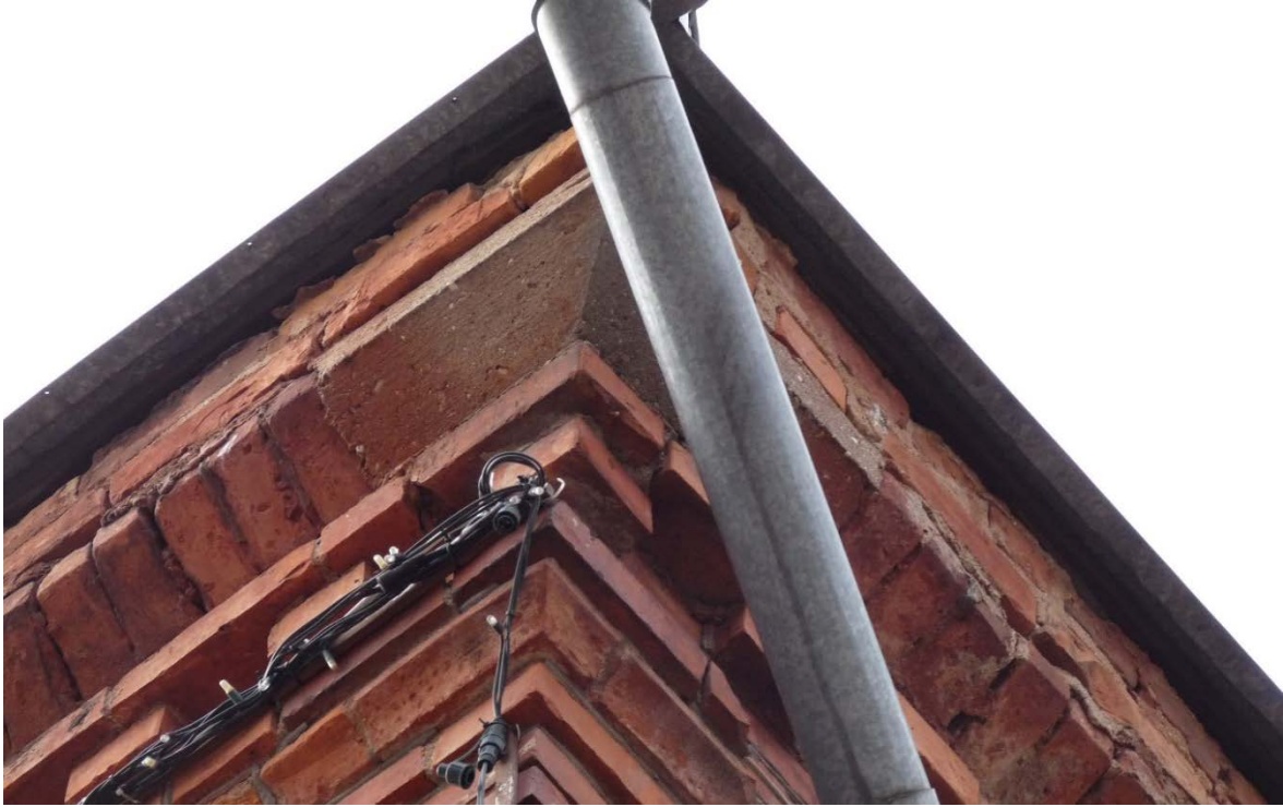
Joonis 37 – Betoonplokiga asendatud nurk – Kaaret, T. 10.04.2015
