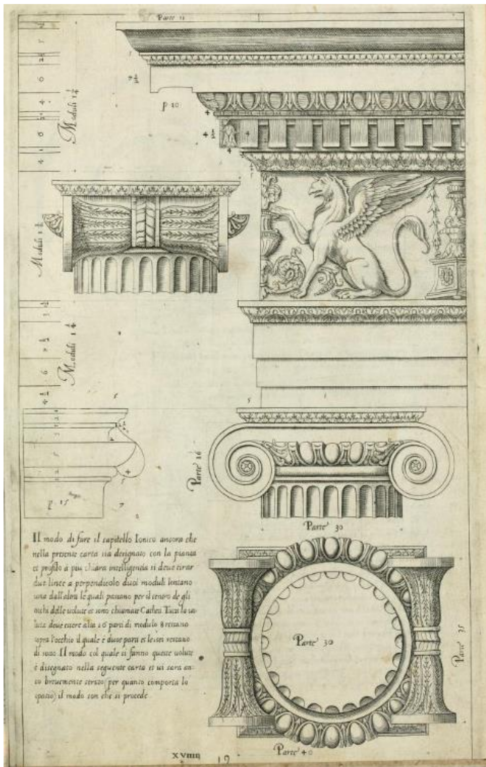
Joonis 91 – Joonia orderi antablemaan ja kapiteel – Vignola, 1635
