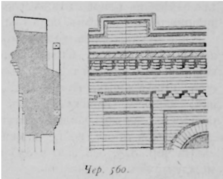
Joonis 23 – Näide saksa telliskarniisiga hoonest – Романовичь, 1903
