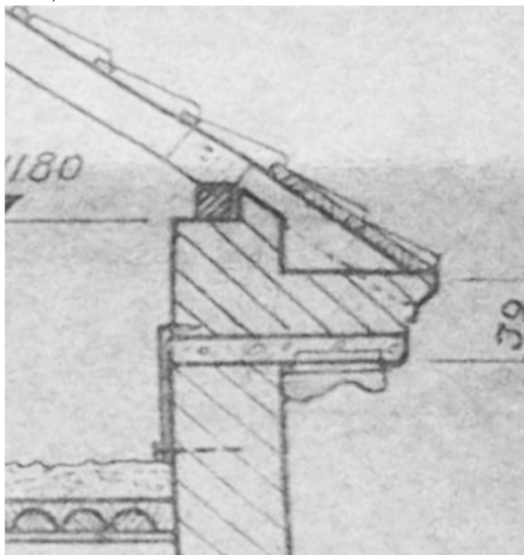
Joonis 75 – Karniisi lõige, 1947 – Idnurm, M. fotokogu
