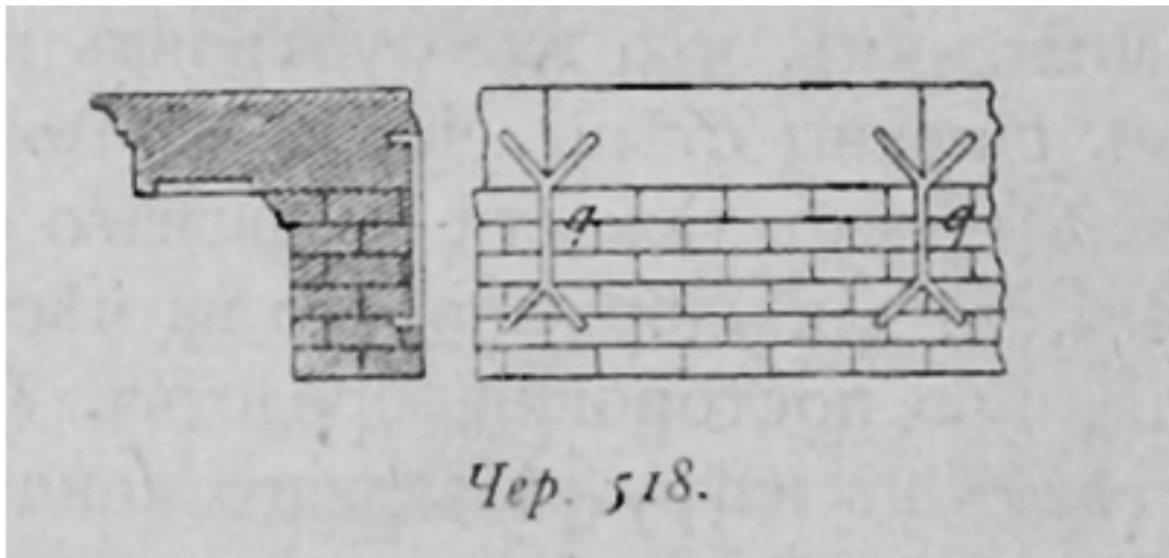
Joonis 21 – Vertikaalsete ankrutega kinnitatud karniis – Романовичъ, 1903
