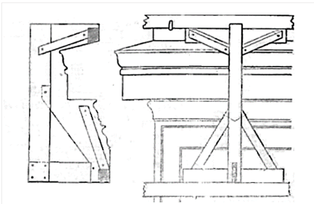
Joonis 40 – Šabloon ja juhtlatid – Романовичь, 1903
