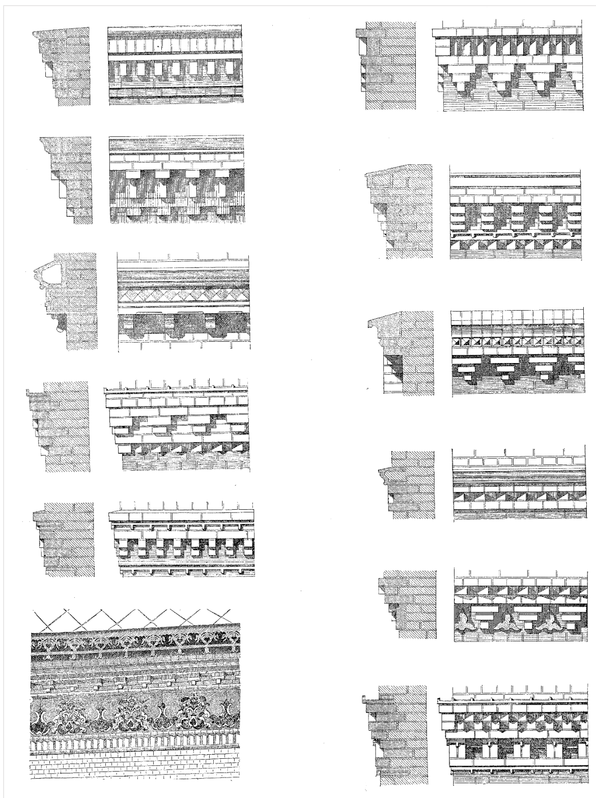
Joonis 25 – Historitsistlikud telliskarniisid – Барановский, 1902–1908
