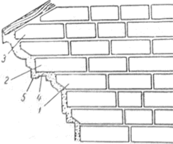
Joonis 3 – Traditsioonilise telliskarniisi osad – Pirogov, N. Ž. (1955). Müürsepa- ja pottsepatööd. Tallinn: Eesti Riiklik Kirjastus.
