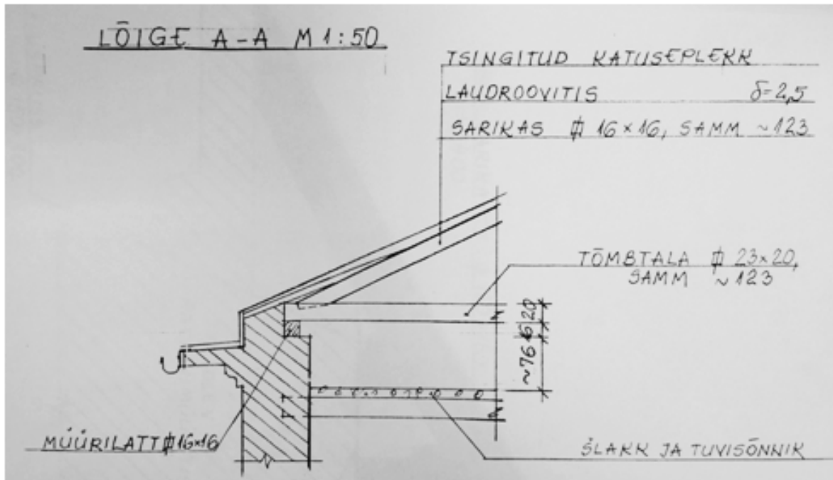
Joonis 66 – Räästasõlme lõige enne rekonstrueerimistöde algust 1998. aastal – Ränd, 1999
