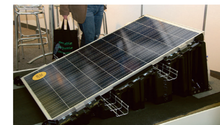
Modi tseeritud bituumenrullmaterjali (MBR) peale MBR lappidega paigaldatav päikesepaneeli alus. Sellise lahenduse kasutamine eeldab katuse kinnituse arvutusi.
